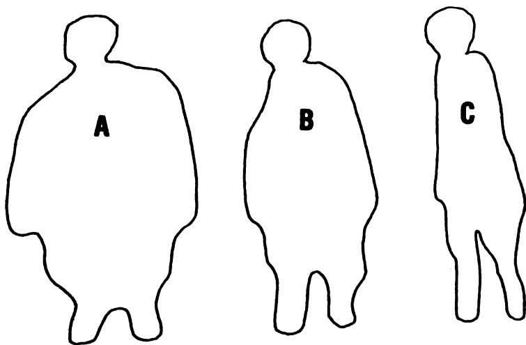
Рис. 4. Диаграмма изменения формы человеческого тела в течение Великого Года.
