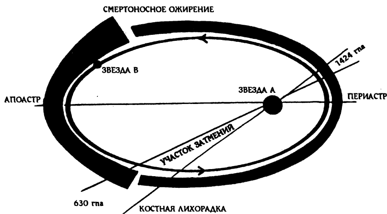
Рис. 5. Диаграмма изменения человеческой биомассы под влиянием гелико-вируса.
