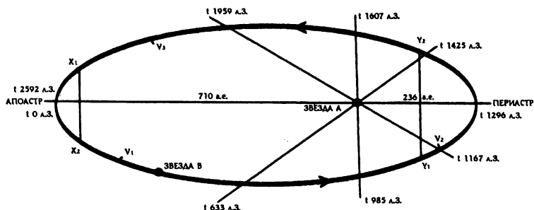
Рис. 2. Орбита
